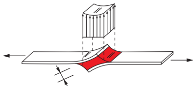
Abb. 1: Größerer Spalt
