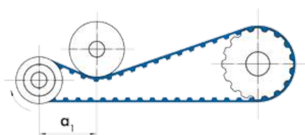
Abbildung 5.1.2: Anordnung der Außenspannrolle
