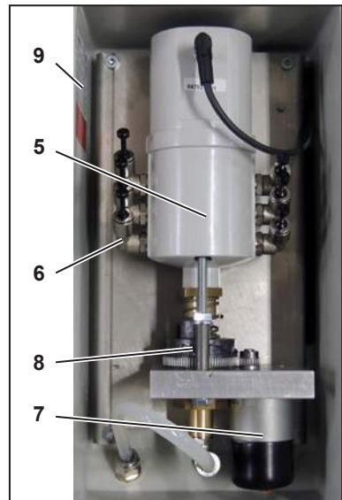
Abb. 3-2 Pumpen- und Verteilereinheit
