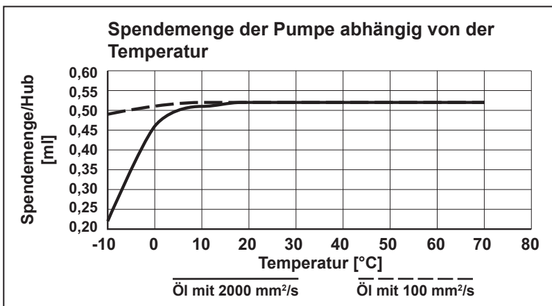
Abb. 9-2 Spendemenge der Pumpe abhängig von der Temperatur
